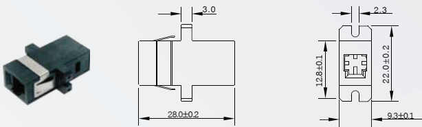
MTRJ SC Footprint Type
